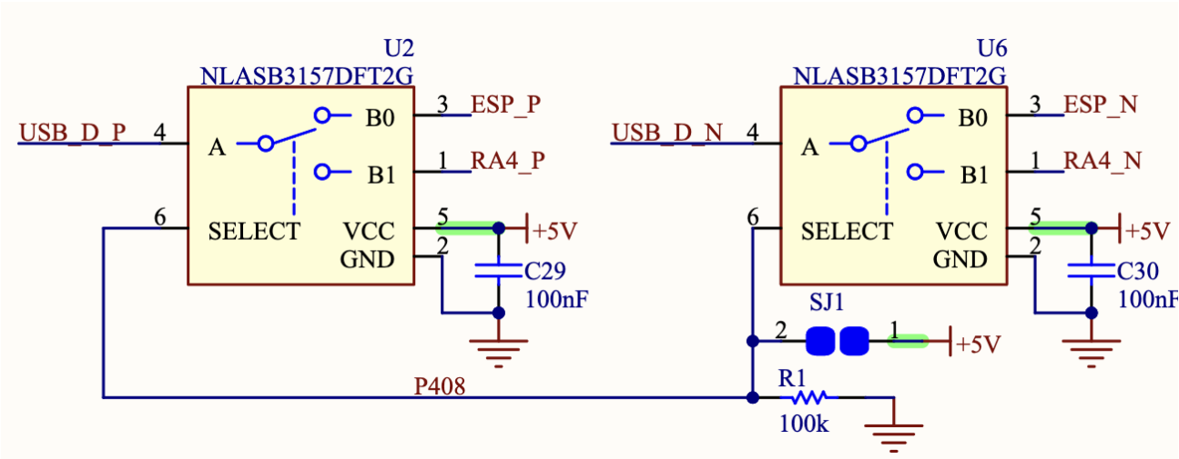
SJ1 是 USB 接口，RA4M1 和 ESP32-S3
